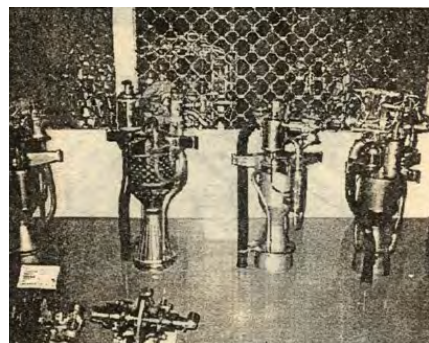
Moteurs S2-711 de l'OKB-2 d'Isaiev
