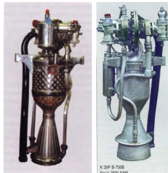
Moteurs S2-711 de l'OKB-2 d'Isaiev
