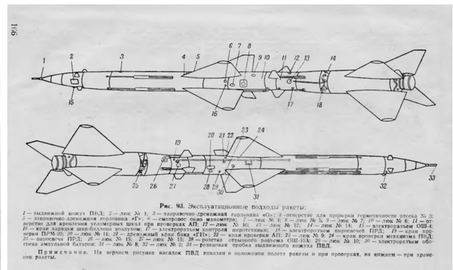
missile V-755 (20D) du système S-75M Volkhov (1961)
