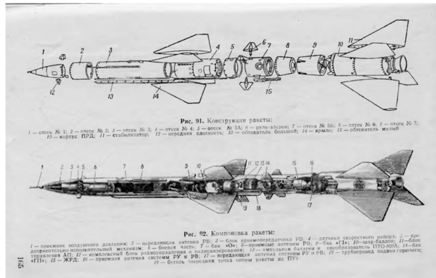
missile V-755 (20D) du système S-75M Volkhov (1961)
