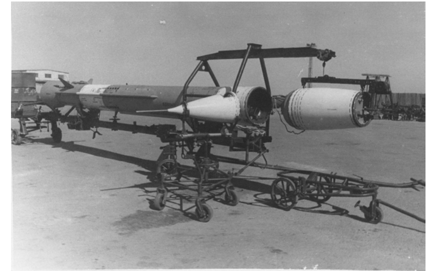
Фото 110. Стыковка изделия РА-6 с ракетой В-760.
